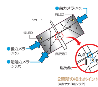
3カメラシステムの構造
