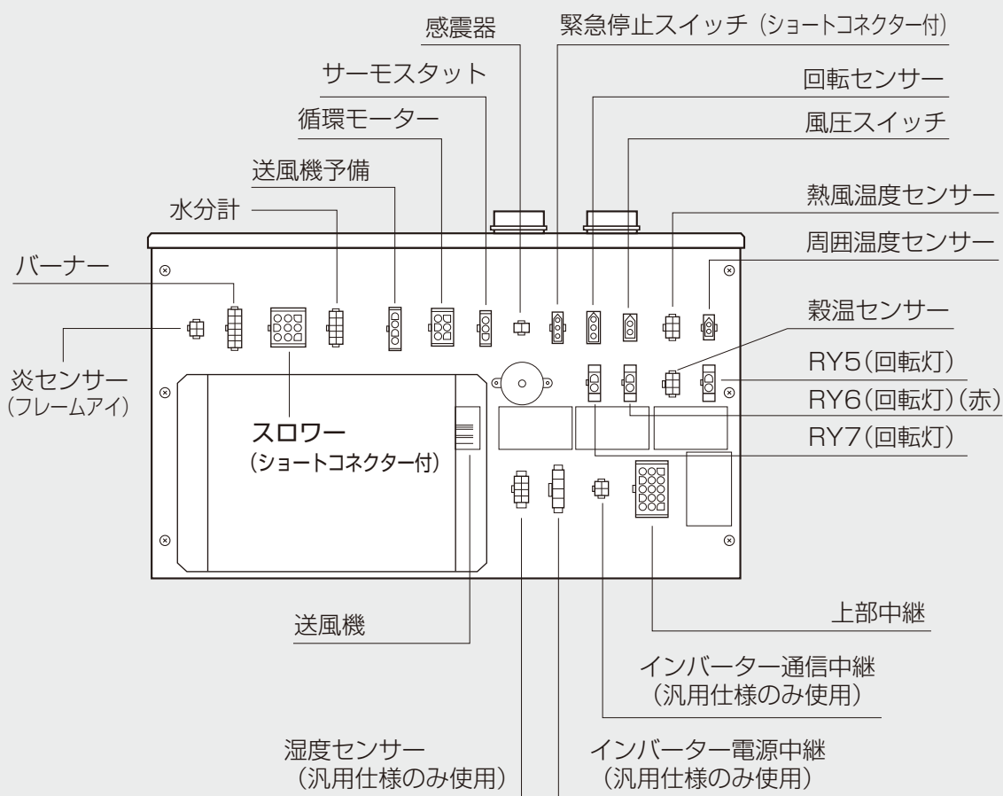
コントロールボックス下面から見たところ
