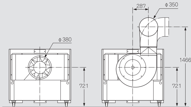
SSE-GSFシリーズ：遠心送風機
