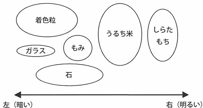
図6-16 反射(まえ、うしろ)カメラによる原料・異物の見え方
