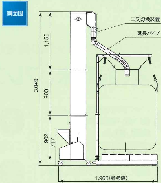
設置寸法 幅×奥行き×高さ(mm) 2,654×1,963×3,049
